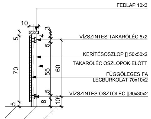
A - A METSZET
