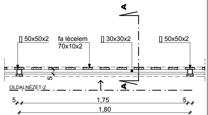
FELÜLNÉZET
