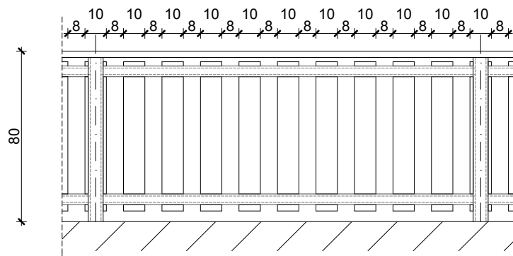
OLDALNÉZET-2
